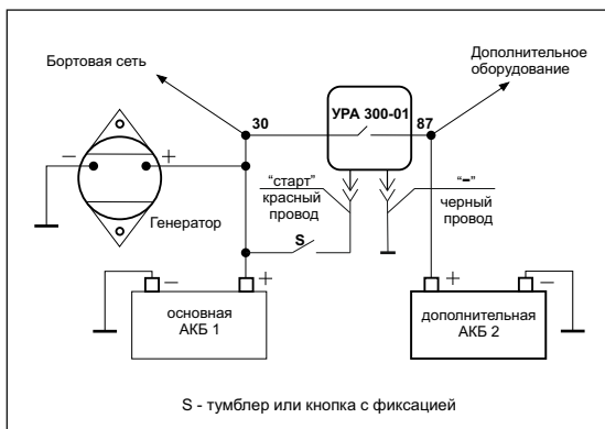
Рис.1. Схема подключения устройства развязки аккумуляторов
